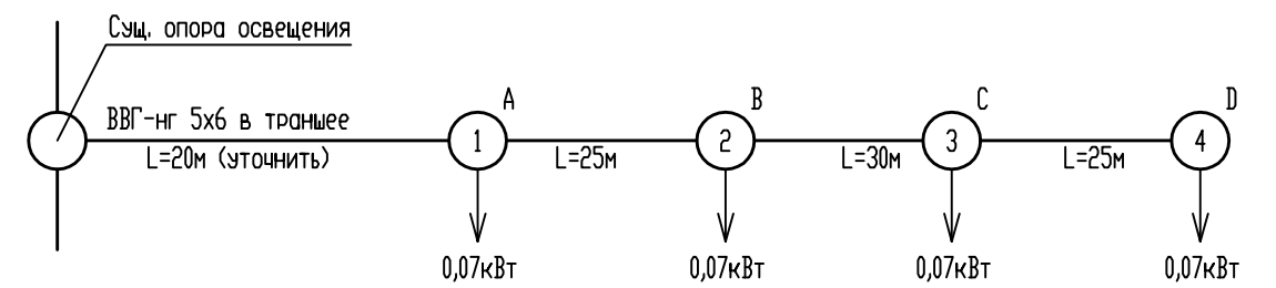
Схема наружного освещения
